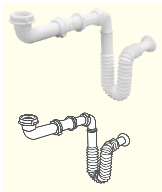
Cespol Ahorrador de Espacio con Cespol Plus XL
